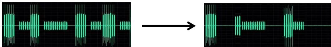
Exemple de déformation de trains rapides de fréquences DTMF
